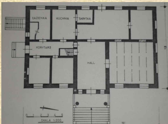
Układ pomieszczeń dworu w Kępczynie (źródło: WUOZ Konin)
