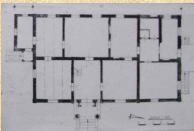
Układ pomieszczeń w dworku w Straszowie (źródło: WUOZ Konin)
