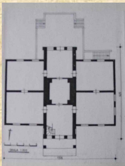
Układ pomieszczeń dworu (źródło:WUOZ Konin)
