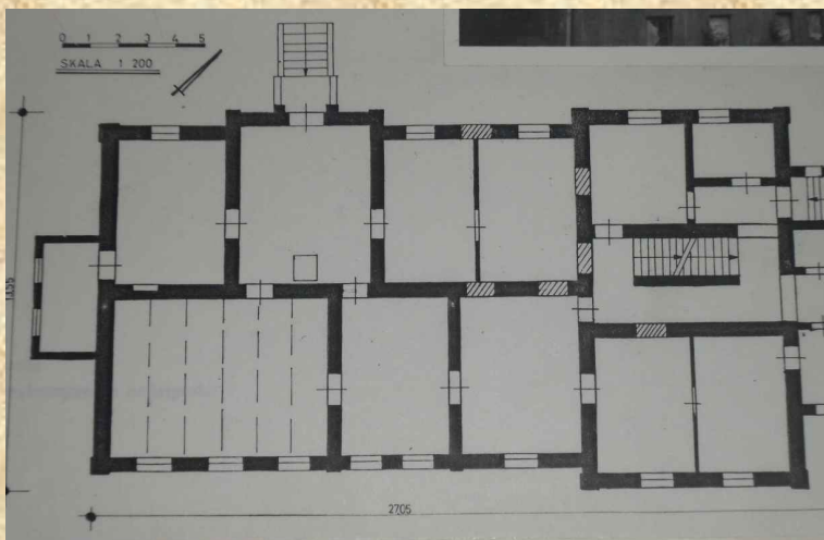
Układ pomieszczeń w dworze w Rgiewie (źródło: WUOZ Konin)
